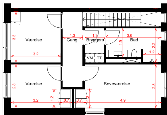
1. sal
