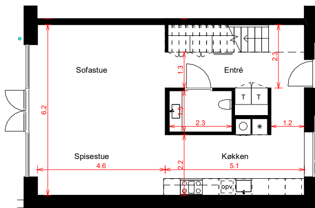
Stueetage
