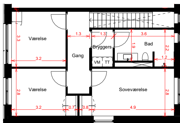
1. sal
