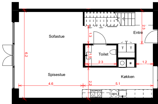
Stueetage
