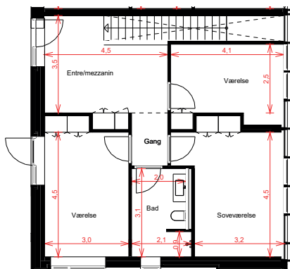
Stueetage
