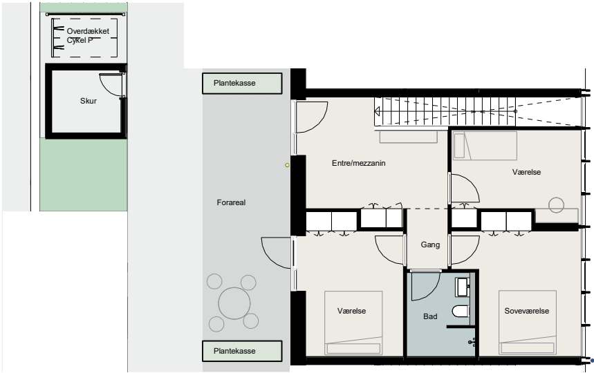
Stueetage
